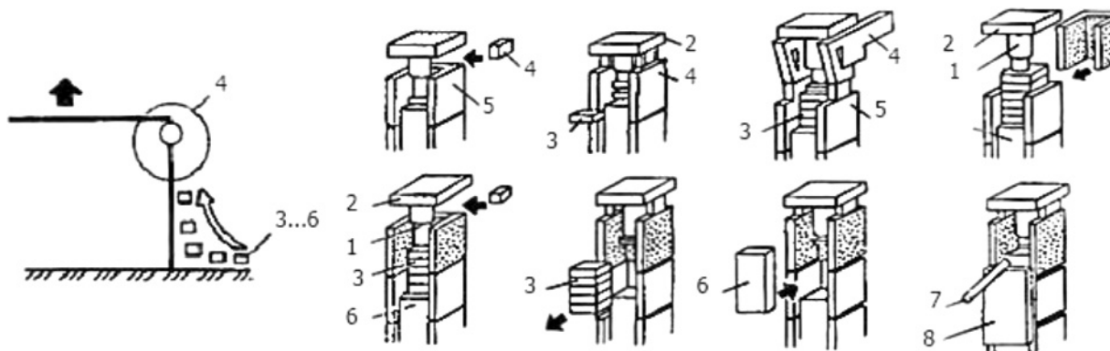
Рис.6 Метод ММ11 – підрощування за допомогою одного домкрата, розташованого в опорних вузлах блоку покриття або на оголовках колони (зростання нижньої частини колони за рахунок нарощування верхньої); 1 – гідродомкрат; 2 – покриття, 3 – центральні прокладки; 4 – бокові прокладки; 5, 6 – відповідно, зовнішні і внутрішні елементи колони; 7 – шланг для нагнітання бетонної суміші; 8 – щит опалубки
