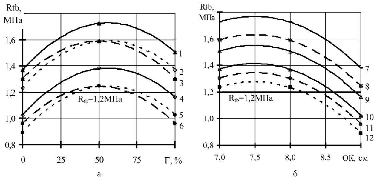
Рис. 1. Залежність міцність на розтяг у разі згину штукатурки: а – від ступеня ґрунтування основи за рухомості 7 см, 8 см, 9 см; б – від рухомості за ґрунтування основи 0%, 50%, 100%: 1 – \omega_m=2,2\% ; ОК=7см, 8 см; 2 – \omega_m=0,6\% ; ОК=7см, 8 см; 3 – \omega_m=1,4\% ; ОК=7см, 8 см; 4 – \omega_m=2,2\% ; ОК=9 см; 5 – \omega_m=0,6\% ; ОК=9см; 6 – \omega_m=1,4\% ; ОК=9см; 7 – \Gamma=50\% \omega_m=2,2\% ; 8 – \Gamma=50\% \omega_m=0,6\% і \Gamma=50\% \omega_m=1,4\% ; 9 – \Gamma=100\% \omega_m=2,2\% ; 10 – \Gamma=0\% \omega_m=2,2\% і \Gamma=100\% \omega_m=0,6\% ; 11 – \Gamma=100\% \omega_m=1,4\% і \Gamma=0\% \omega_m=1,4\% ; 12 – \Gamma=0\% \omega_m=0,6\%
