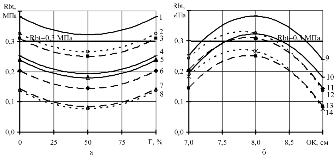
Рис. 2. Залежність міцність зчеплення штукатурки з основою: а – від ступеня ґрунтування основи за рухомості 7 см, 8 см, 9 см; б – від рухомості за ґрунтування основи 0%, 50%, 100%: 1 – \omega_m = 2,2\% ; ОК= 8 см; 2 – \omega_m = 0,6\% ; ОК= 8 см; 3 – \omega_m = 1,4\% ; ОК= 8 см; 4 – \omega_m = 2,2\% ; ОК=7 см; 5 – \omega_m = 0,6\% ; ОК=7см і \omega_m = 2,2\% ; ОК=9 см; 6 – \omega_m = 1,4\% ; ОК=7см; 7 – \omega_m = 1,4\% ; ОК=9см; 8 – \omega_m = 0,6\% ; ОК=9см; 9 – \Gamma = 100\% і \Gamma = 0\% за \omega_m = 2,2\% ; 10 – \Gamma = 50\% \omega_m = 2,2\% ; 11 – \Gamma = 0\% і \Gamma = 100\% за \omega_m = 1,4\% ; 12 – \Gamma = 0\% і \Gamma = 100\% за \omega_m = 0,6\% ; 13 – \Gamma = 50\% \omega_m = 1,4\% ; 14 – \Gamma = 50\% \omega_m = 0,6\%
