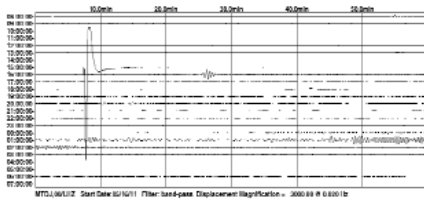
Рисунок 4. Скачок геодеформацій
