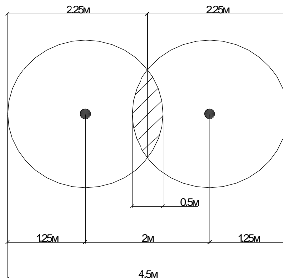
Рис.2. Схематическое изображение распространения инъекционного раствора от инъектора при шаге скважин 2м
