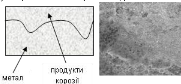
Рис. 5. Нерівномірна корозія
